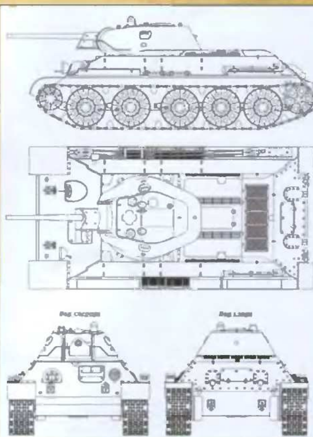
Т-34 выпуска 1942 года. Сталинградский завод № 183.
