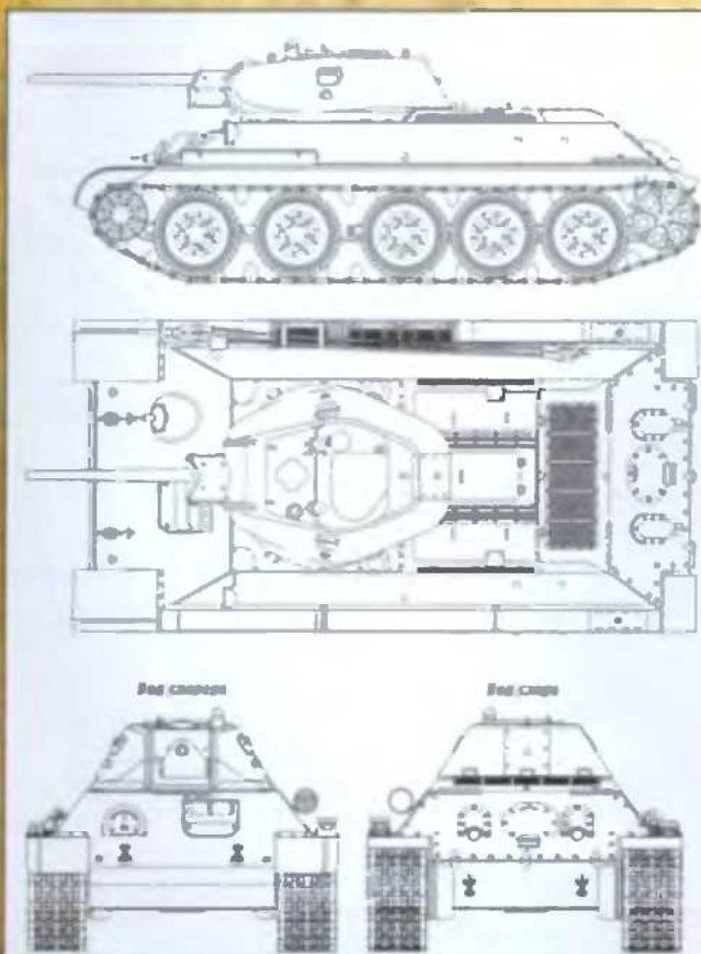
Т-34 выпуска 1942 года. Завод № 183.
